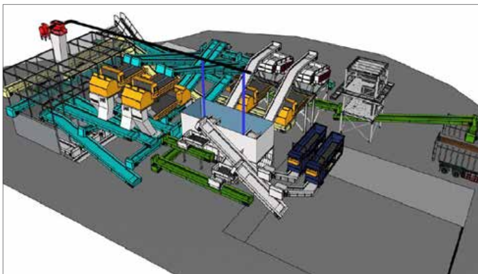
הדמיית מתקן למיון פסולת אריזות
