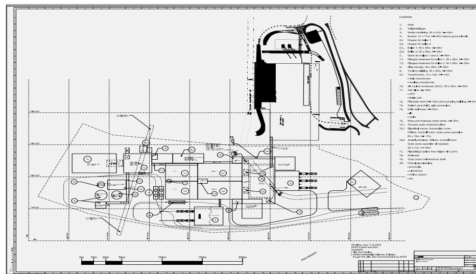
תכנית העמדה ראשונית מתקן השבת פסולת לאנרגיה
